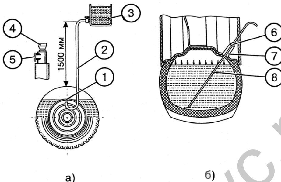
Схема наполнения камер колес жидкостью (а) и удаление жидкости из колес (б):
