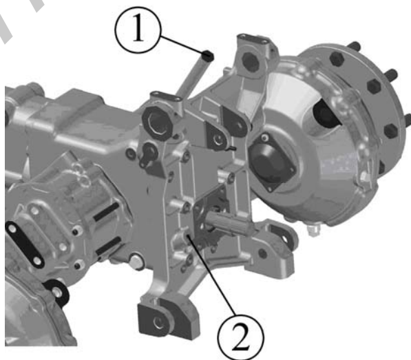
1 – заливная горловина заднего моста; 2 – пробка контрольного отверстия;
